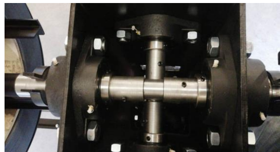
Innenansicht des Turms von oben
