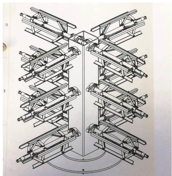
Ausführung mit 12 Stationen
