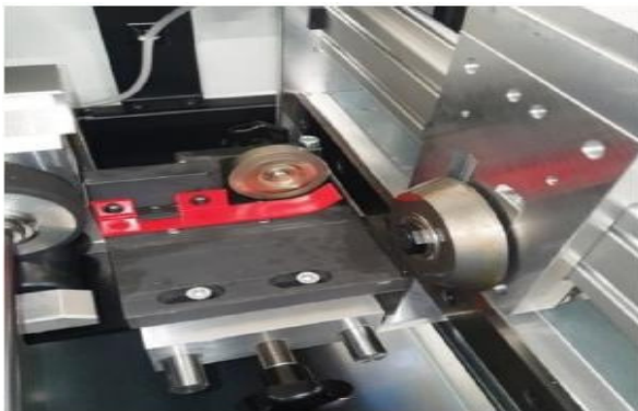
Einlauf (Blecheinzug) von vorn
