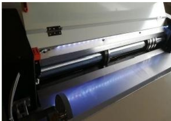
Sicherheitsschalter der Messerwellenhaube
