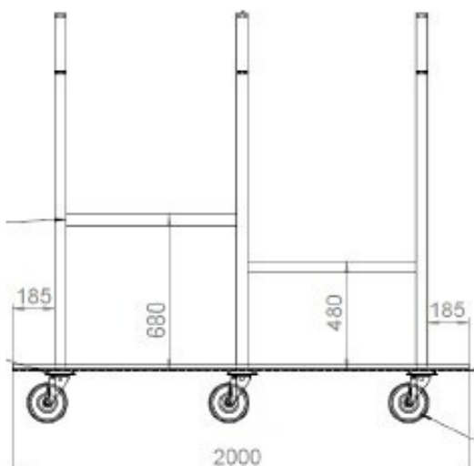
Fächer- / Sektionsmaße
