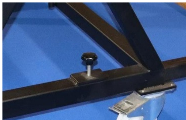
Klemmbremse
