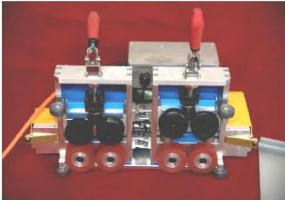
Kompletter Rollensatz (Profilier Rollen gehärtet)
