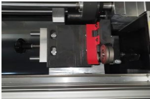
Längsschneideeinrichtung (zusätzlicher Zuschnitt der Bleche möglich)
