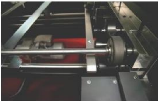
Abgesicherte Schubladenführung für händischen Eingriff
