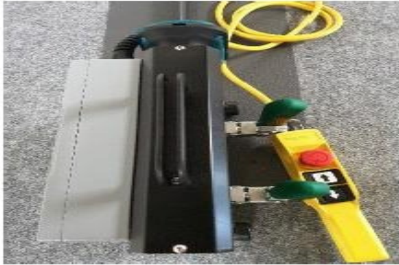
Makita Akku-Anschluss
