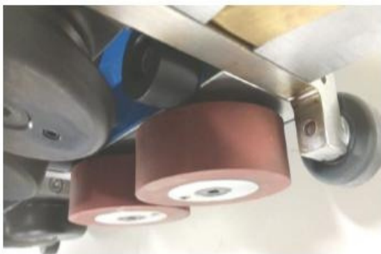
Konkav- und Konvex- Einstellung der Maschine (mittels Druckknopfs)
