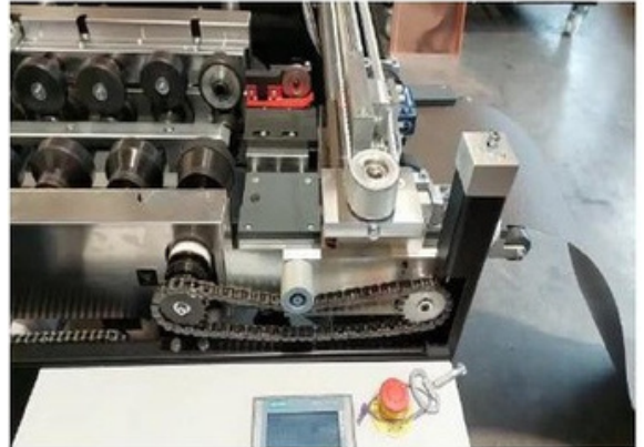
Steuerungsdisplay, Starttaste und Notausschalter
