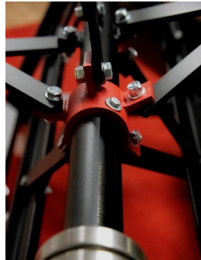
Spindel zum Verstellen des Spreizdorns
