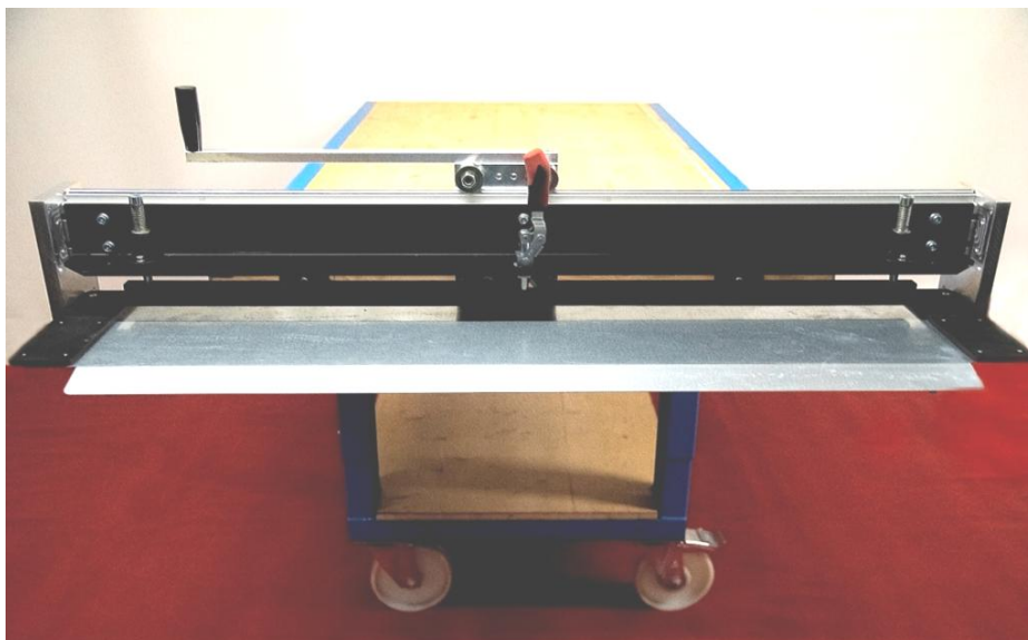
Zuschneid- und Ablängttisch optional mit Handschere TS 1000 oder TS1250mm
