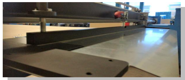
Handschere mit Niederhalter (gummiert) und Obermesser mit integrierter Führungsrolle
