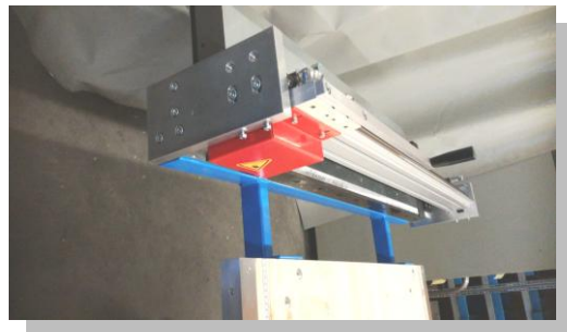
Integrierte Handschere (1000-1300mm) abklappbar, falls nicht benötigt
